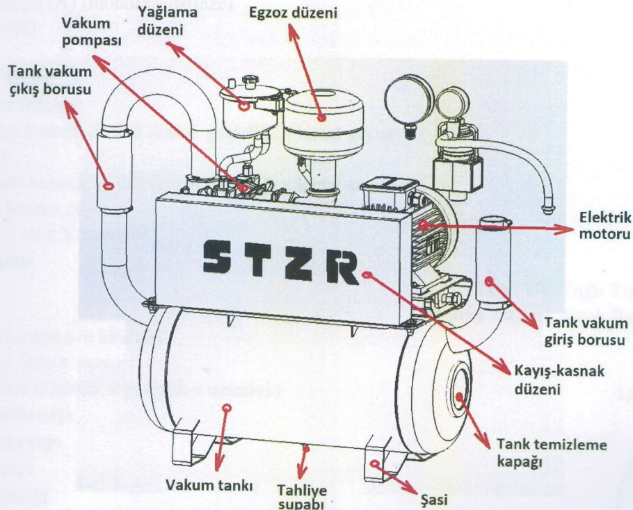
Şekil 3. Vakum üretme grubu önemli kısımları
