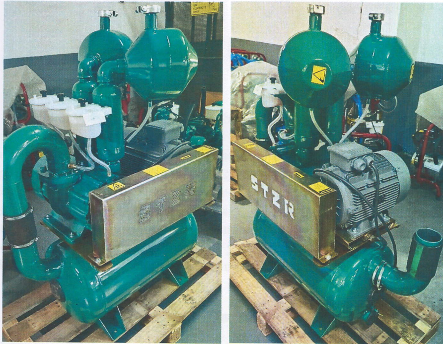
Şekil 1. Sağım sisteminin vakum üretme grubu
