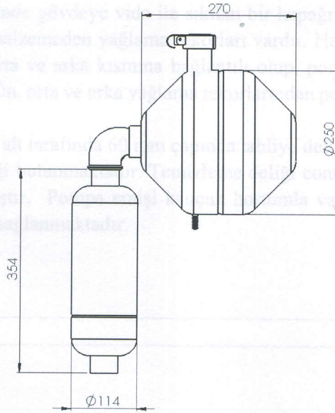
Şekil 2. Vakum üretme grubunun bir egzoz sisteminin genel ölçüleri
